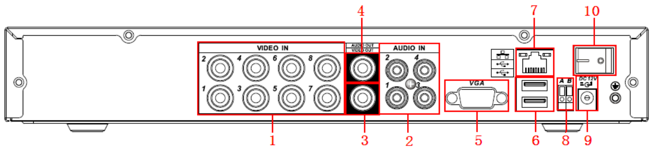
Rysunek 2-2b. Wygląd tylnego panelu rejestratora 8-kanalowego.
