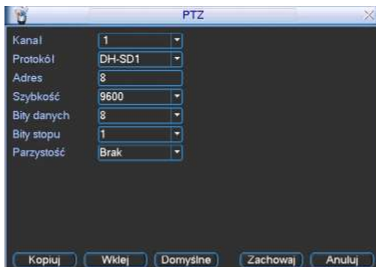
Rys. 4-19. Ustawienia PTZ.
