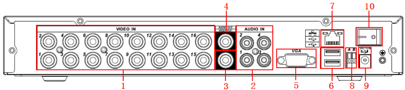
Rysunek 2-2c. Wygląd tylnego panelu rejestratora 16-kanalowego.
