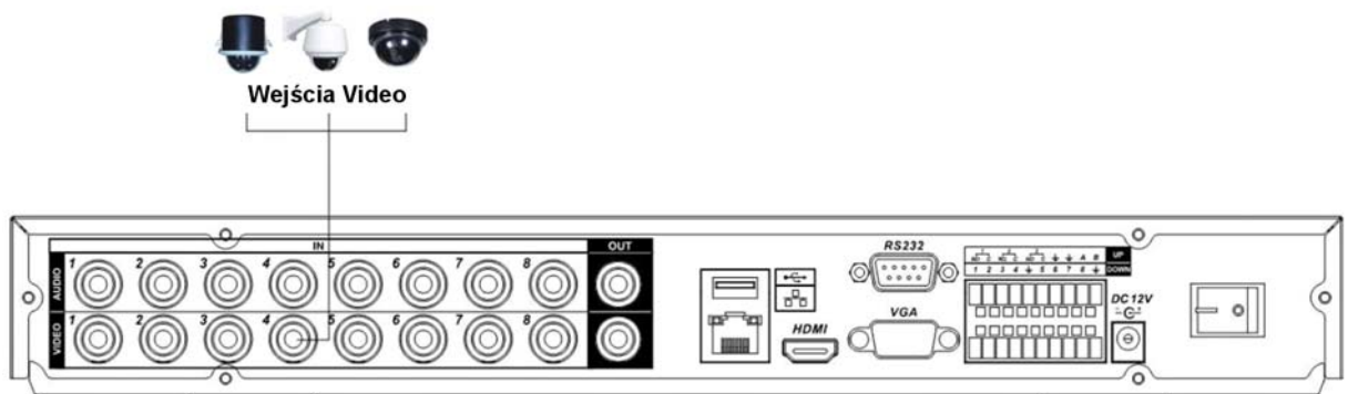
Rys. 3-1. Podłączenie kamer do rejestratora.
