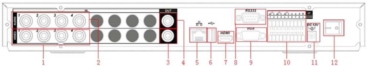
Rysunek 2-2a. Widok tylnego panela rejestratora 4-kanalowego serii LE-A.
