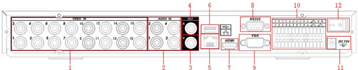
Rysunek 2-2c. Widok tylnego panela rejestratora 16-kanalowego serii LE-A.
