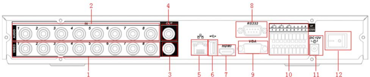
Rysunek 2-2b. Widok tylnego panela rejestratora 8-kanalowego serii LE-A.
